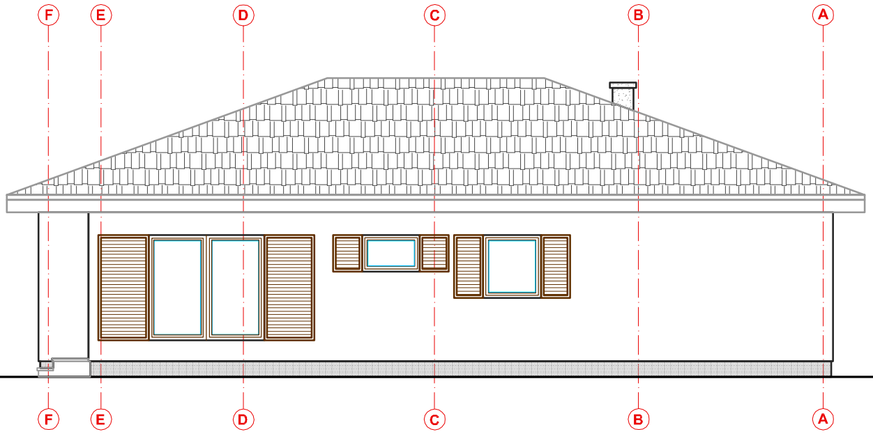
ZAPADNA FASADA
