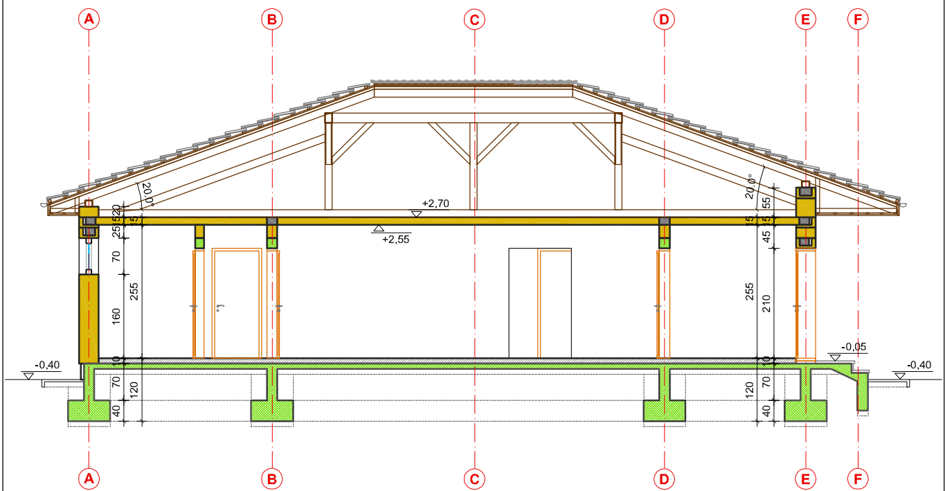
PRESEK 2-2
