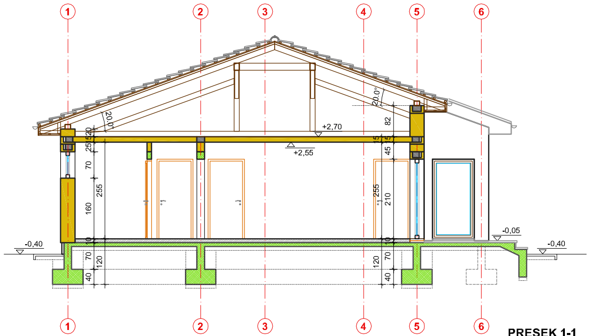
PRESEK 1-1
