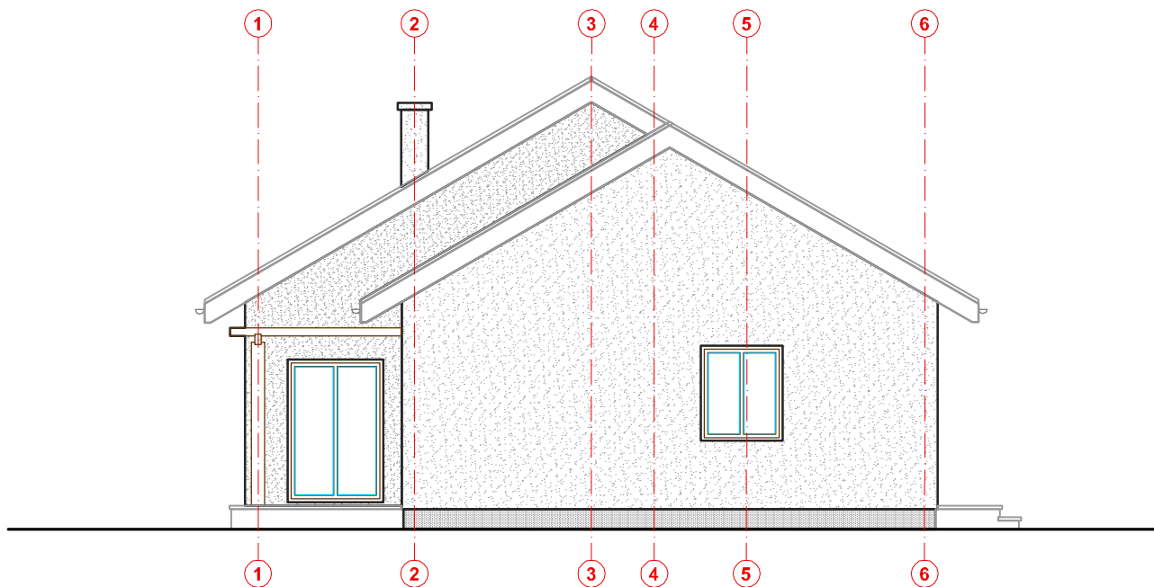
JUŽNA FASADA
