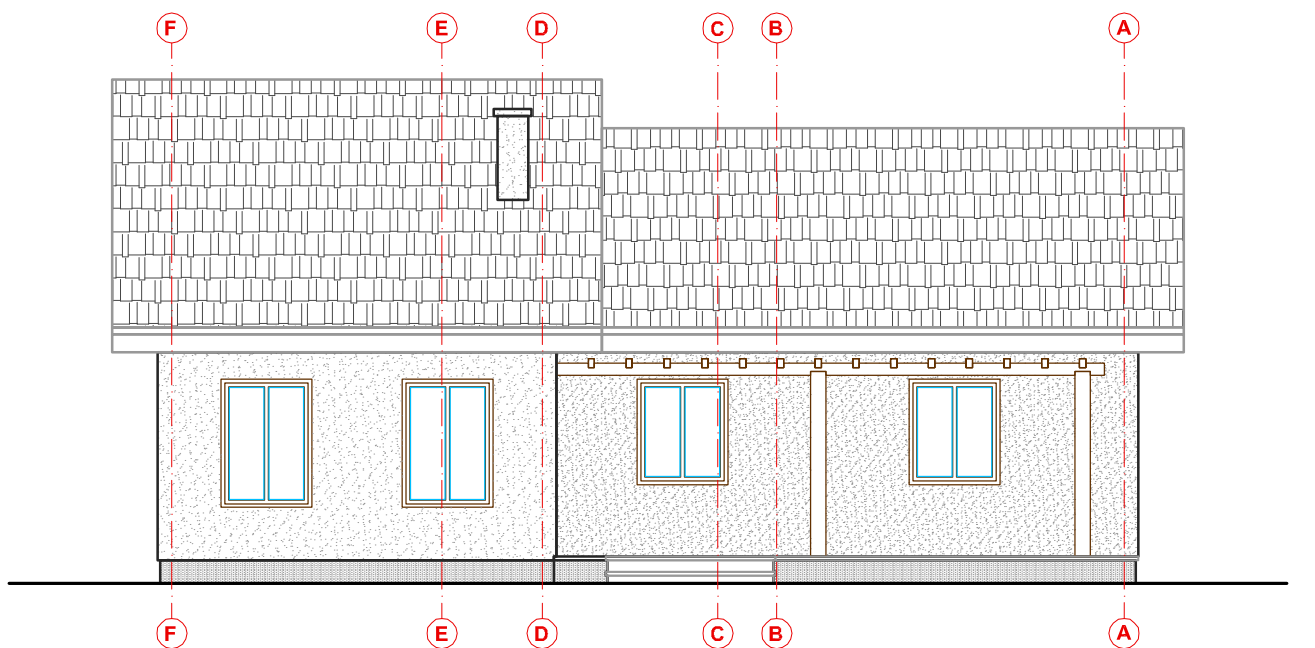
ZAPADNA FASADA
