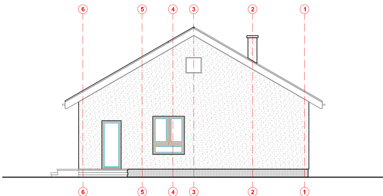
SEVERNA FASADA
