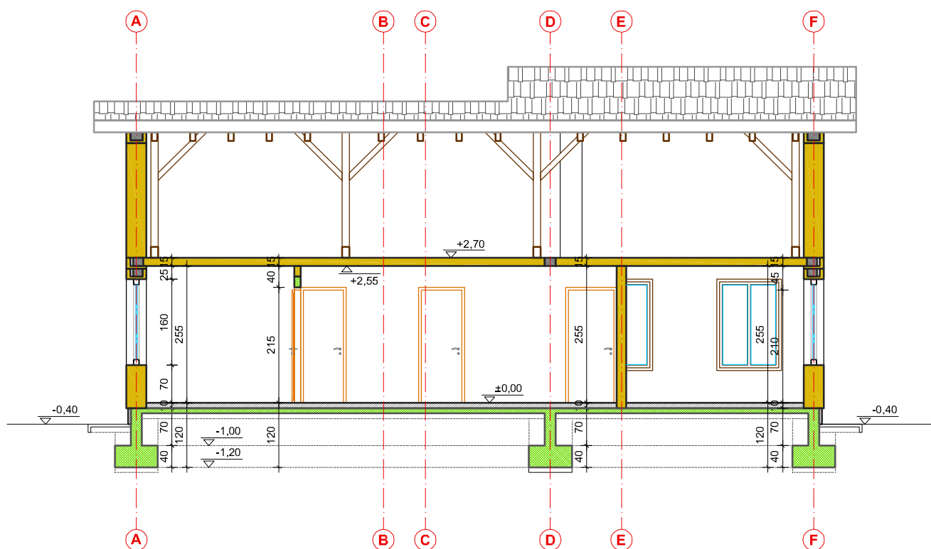
PRESEK 3-3
